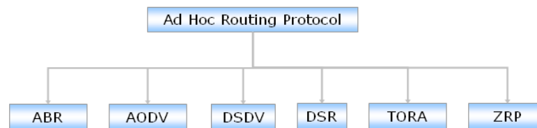
Figure 2: Πρωτόκολλα Δρομολόγησης
